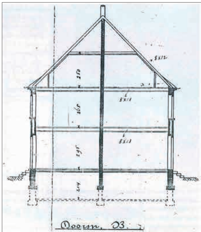
Doorsnedetekening van twee Helmathuizen.
